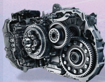
Hộp số tự động 6 cấp (EAT6)
